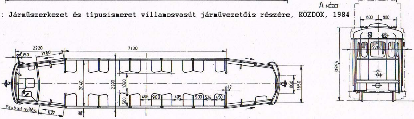
7.1. ábra 1500-as pályaszámú motorkocsik jellegrajza és fontosabb villamos berendezéseinek elhelyezése
