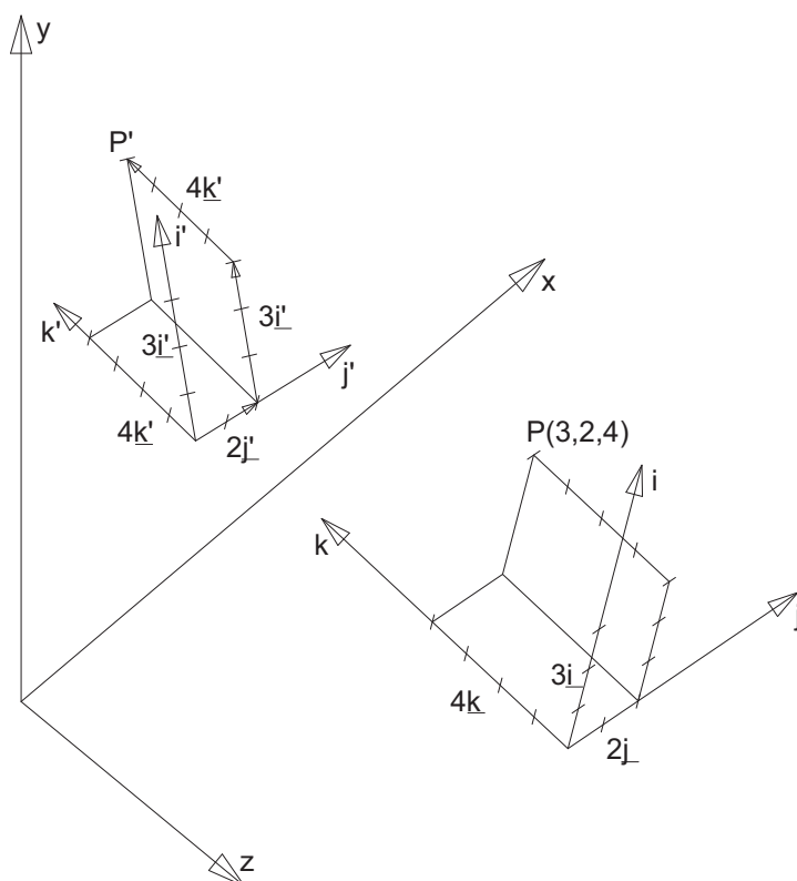
3. ábra. P pont axonometrikus képe
