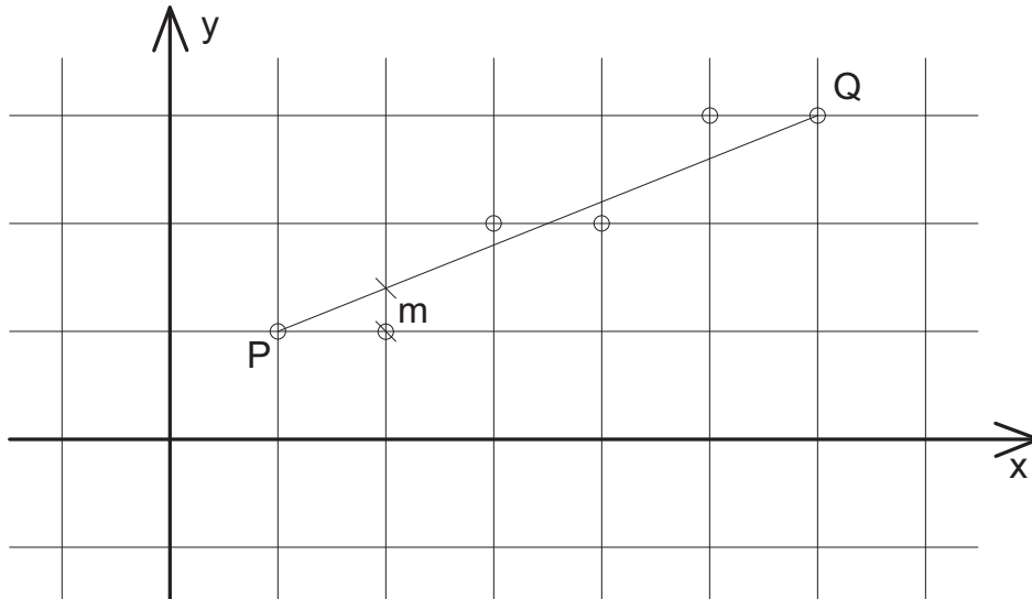
1. ábra. Szakasz rajzolása a raszteres képernyőn
