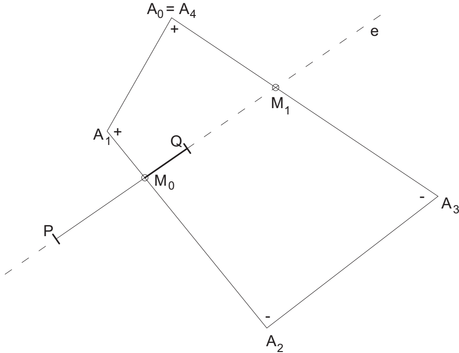
4. ábra. Szakasz vágása konvex sokszögre
