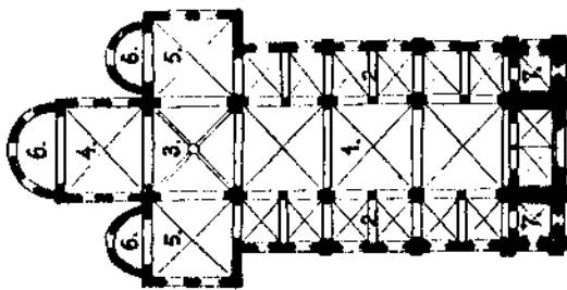
HÁROMHAJÓS ROMÁN BAZILIKA
