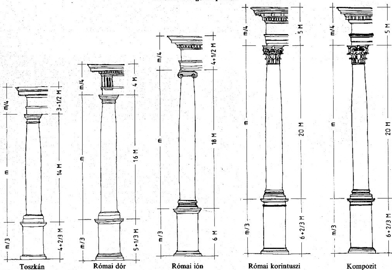
11. ábra. Római oszloprendek
