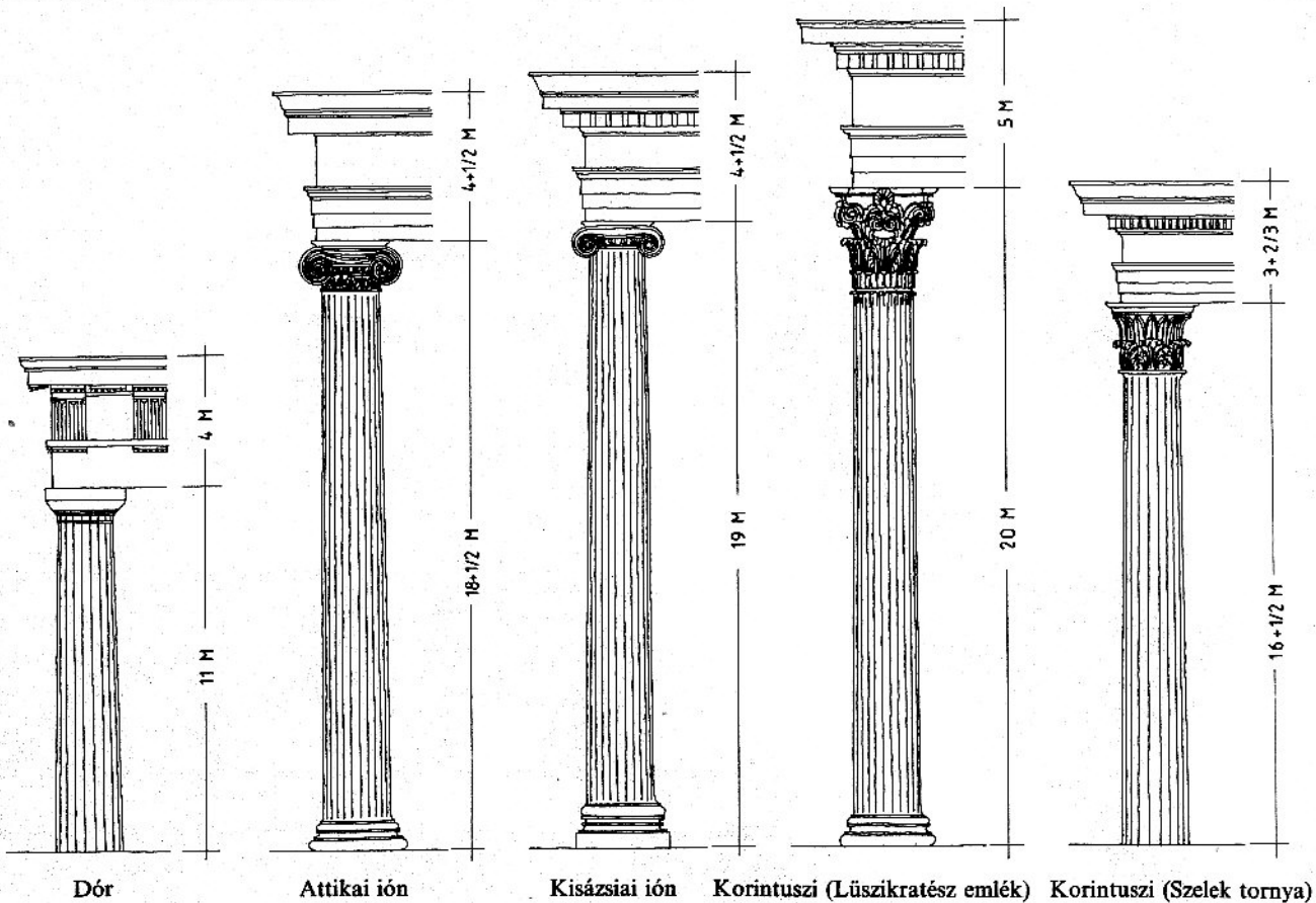
10. ábra. Görög oszloprendek
