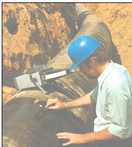
1.24. ábra Földalatti csővezeték varratának helyszíni ultrahagos vizsgálata
