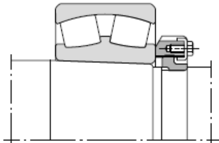
14.7 Ábra Osztott menetes gyűrűvel történő rögzítés
