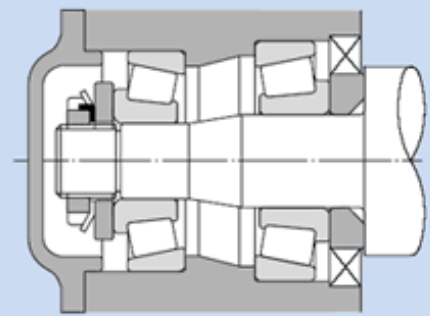
15.9 Ábra Az axiális játék beállítása csapágyanya segítségével
