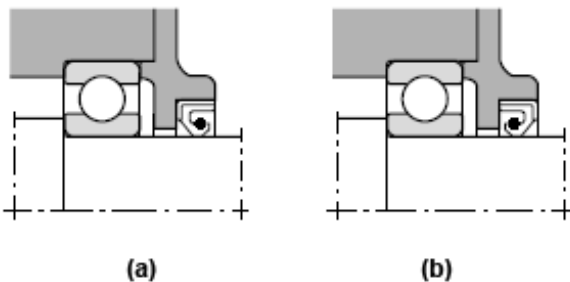
12.11 Ábra Olajtömítések
