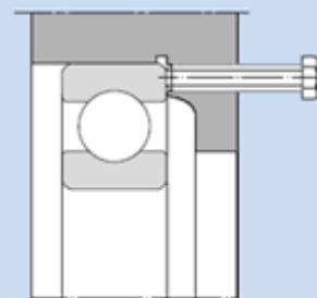
15.16 Ábra Mentés furat alkalmazása a kiszereelés megkönnyítése céljából
