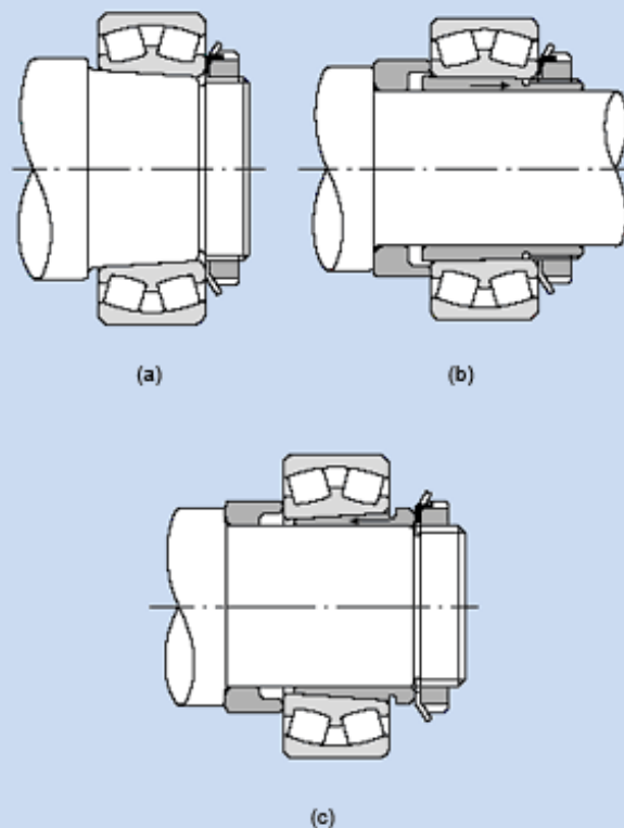
15.5 Ábra Beépítés állítónya alkalmazásával
