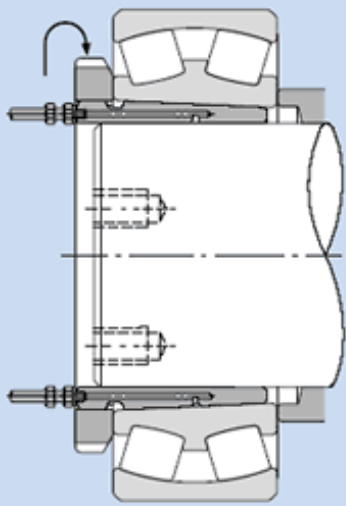
15.22 Ábra Hidraulikus hüvellyel történő csapágykiszereles
