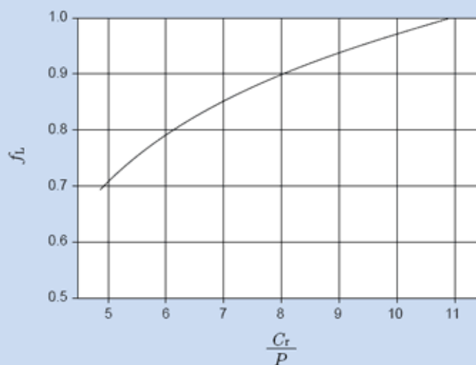
9.1 Ábra Terhelési tényező f_L C/P -től függően
