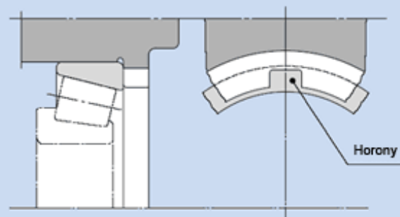
15.15 Ábra Kikönyvítés kimarása a házban kiszereelés elősegítésére
