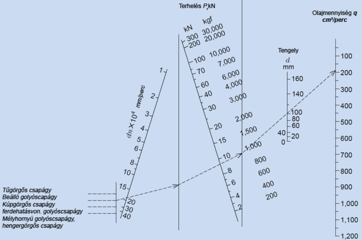
11.12 Ábra A szükséges olajmennyiség megállapítása becslés alapján
