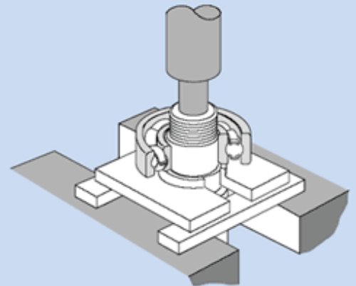
15.13 Ábra Kiszereles prés alkalmazásával
