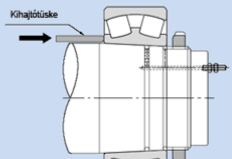
15.19 Ábra Kiszereles lehúzóhüvely segítségével
