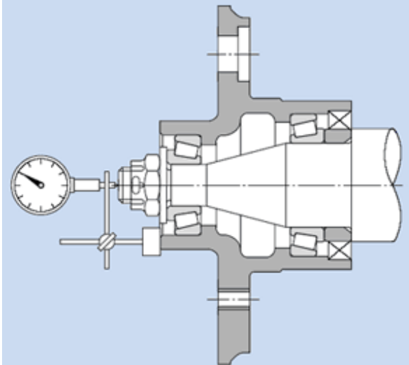
15.10 Ábra Az axiális játék beállítása mérőóra felhasználásával
