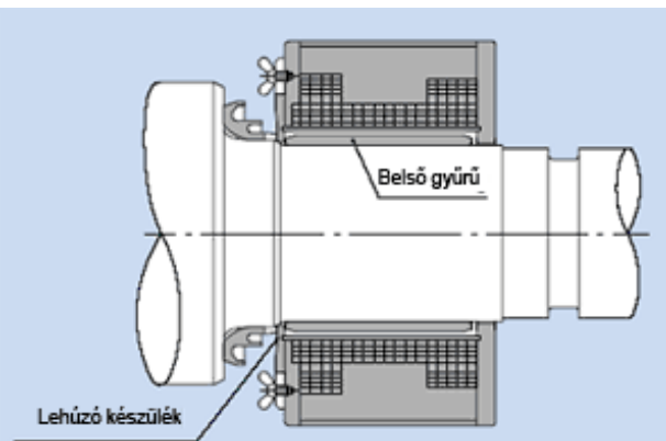
15.4 Ábra Indukciós tekercessel ellátott elektromos lehúzó készülék
