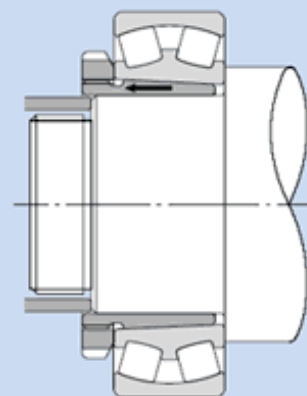
15.19 Ábra Kiszereles lehúzóhüvely segítségével
