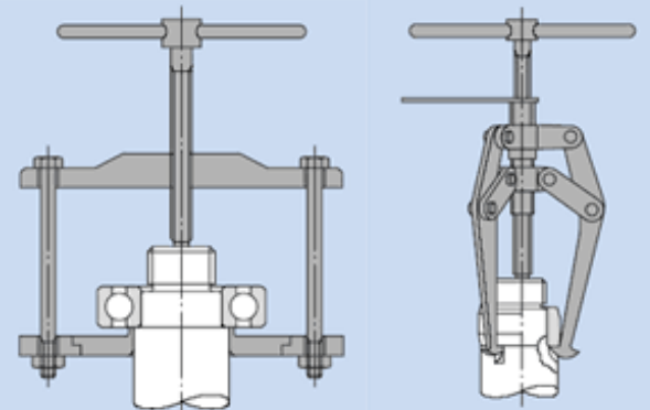
15.12 Ábra Lehúzókészülék
