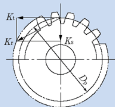
6.3 Ábra Kiadódó radiális erők
