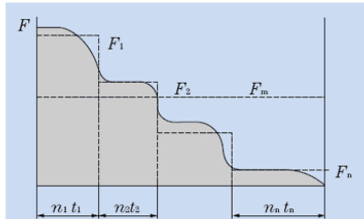
6.8 Ábra Lépcsős terhelésváltozások
