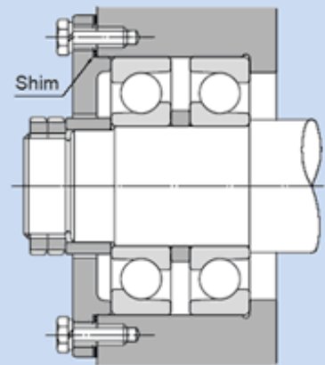
15.11 Ábra Az axiális játék beállítása alátétárcsa alkalmazásán keresztül
