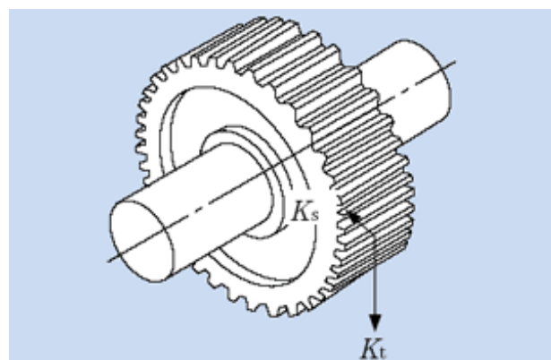
6.1 Ábra Erőhatások egyenes fogazású homlokkeréken
