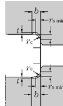
14.8 Ábra Közvetétygyűrűk
