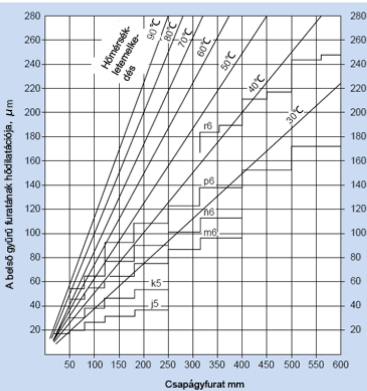
15.3 Ábra A tőrésátfedés miatt szükséges hőmérsékletkülönbségek
