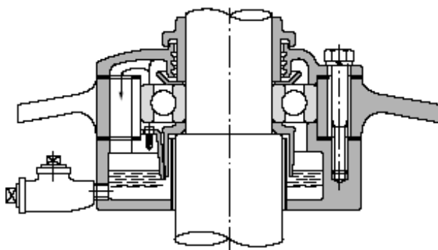
11.3 Ábra Szóróolajkenés
