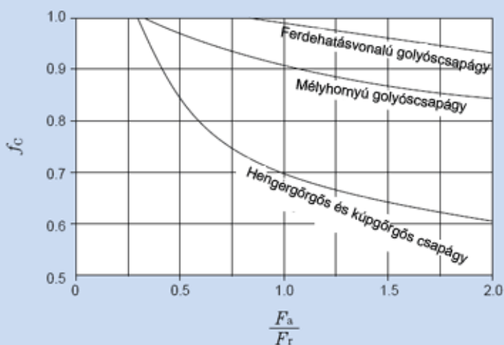
9.2 Ábra Terhelési tényező f_c F_a/F_r -től
