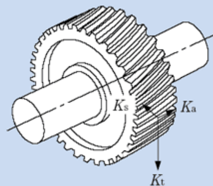
6.2 Ábra Erőhatások ferdefogazású homlokkeréken
