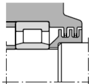
12.5 Ábra Radiális labirint-tömítés
