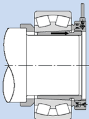
(b) Hidraulikus anya és lehúzóhüvely 15.21 Ábra Hidraulikus anyával végzett kiszereelés
