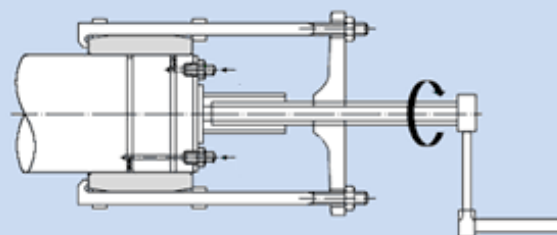
15.17 Ábra Csapágykiszereelés hidraulikus eljárással
