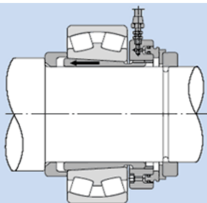
(a) Hidraulikus anya és szorítóhüvely
