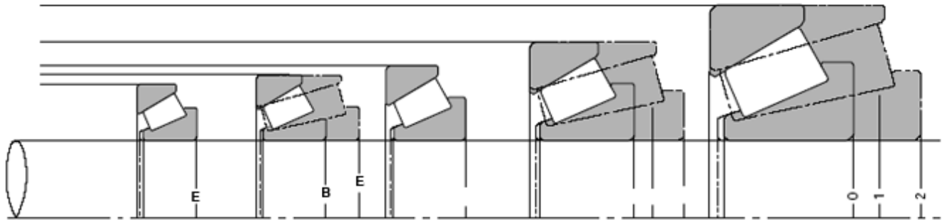
3.6 Ábra Kúpgörgős csapágyak méretsorainak összehasonlítása
