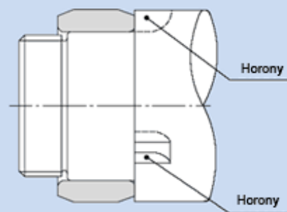
15.14 Ábra Hornyos kikönyvítés a kiszereelés elősegítésére
