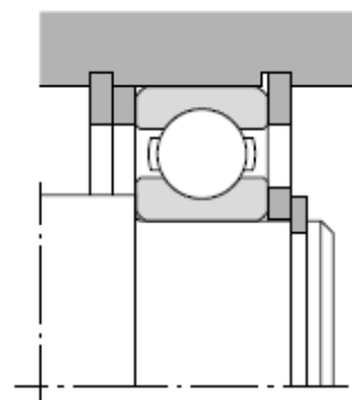
14.3 Ábra Rúgósgyűrűvel történő csapágyrögzítés a tengelyen
