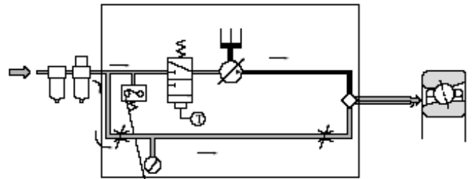
11.9 Ábra Olaj-levegő kenés
