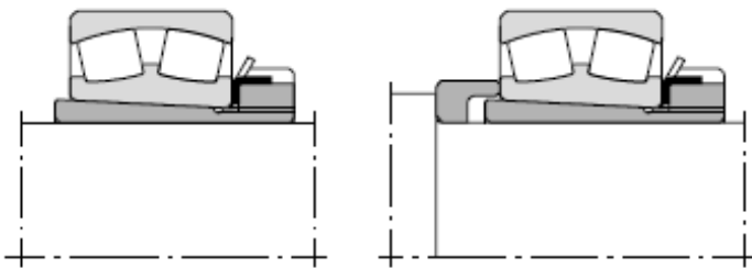
14.5 Ábra Szorítóhüvelyes rögzítés
