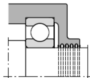
12.2 Ábra Réstömítés
