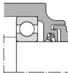
12.9 Ábra Filctömítés Z-profillal
