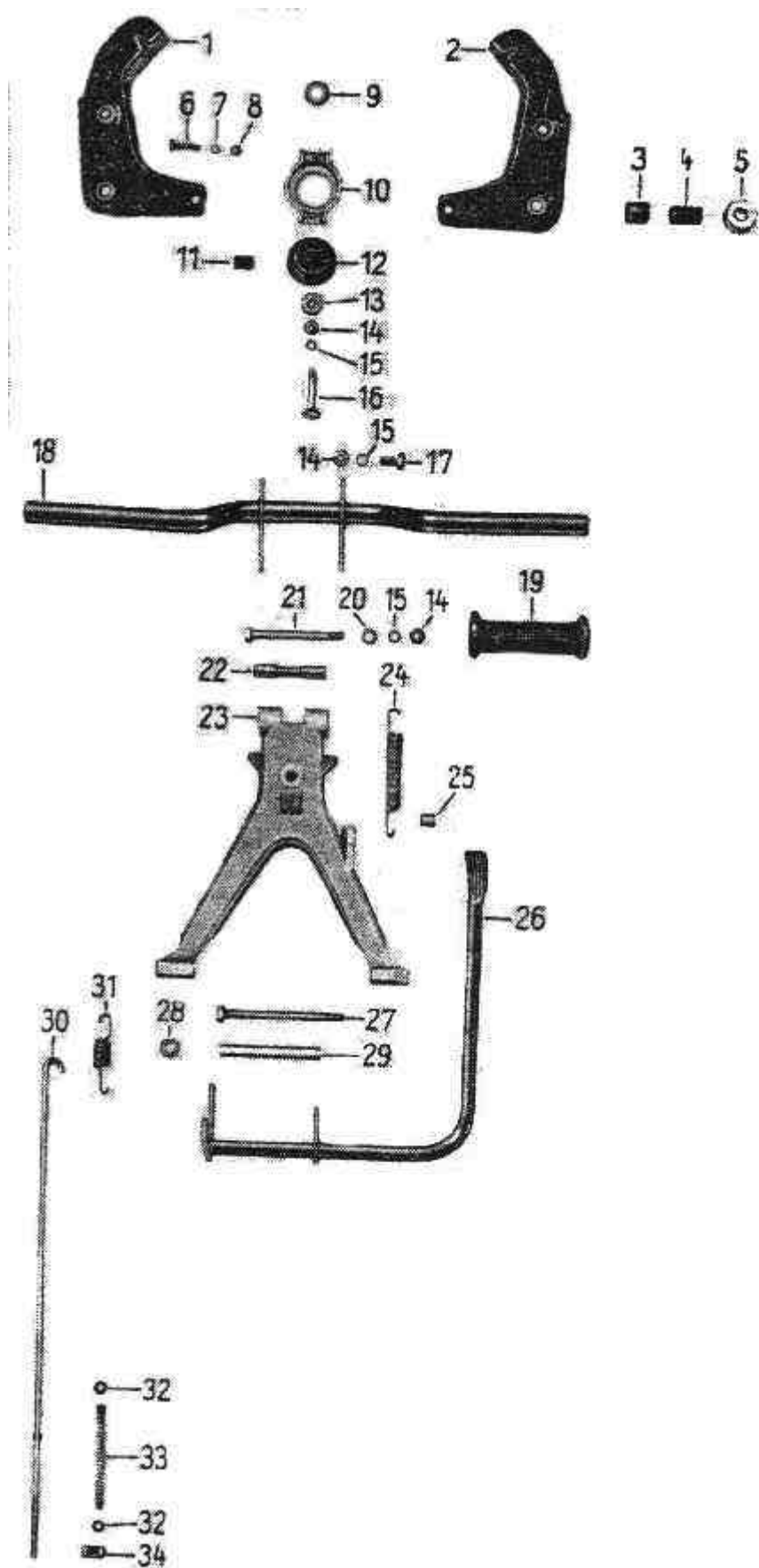
LÁBTARTÓ, MOTORÁLLVÁNY, LÁBFÉKKAR
