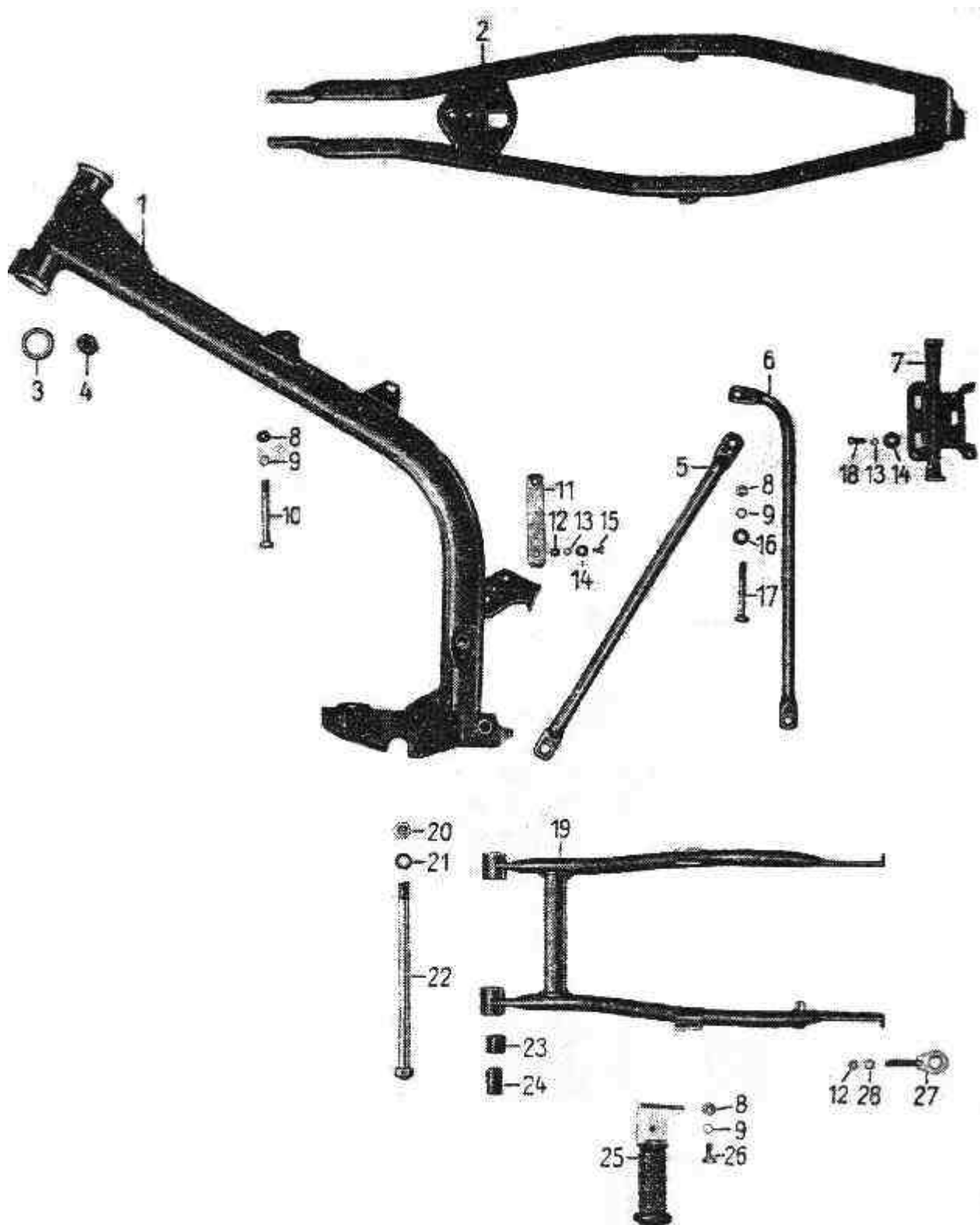
VÁZ, HÁTSÓ LENGŐVILLA
