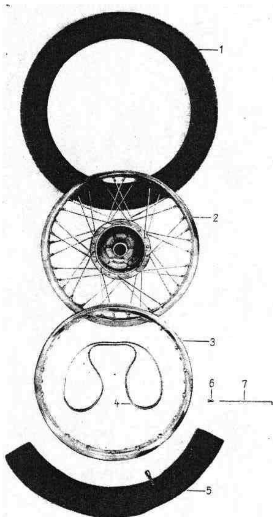
ELSŐ ÉS HÁTSÓ KERÉK
