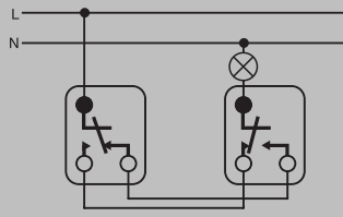
Váltó, alternatív kapcsolás
