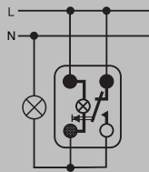
Nyomó külön megvilágítással
