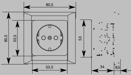
Földelt csatlakozó aljzat
