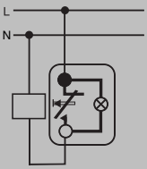
Megvilágított nyomó
