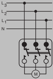
Hárompólusú kapcsoló
