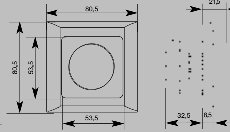
Forgatógombos fényerőszabályzó
