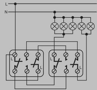
Kettős dupla alternatív kapcsolás
