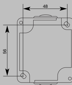
Felfogatócsavarok közötti távolság
