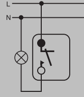
Egypólusú kapcsoló
