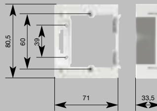
Kiemelő sorolókeret
