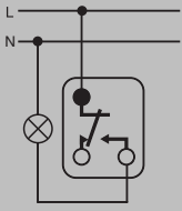
101-es kapcsoló
