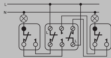
Kettős alternatív kapcsolás
