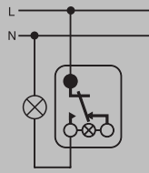
101-es kapcsoló mint egypólusú, megvilágított
