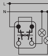
2-pólusú nyomó
