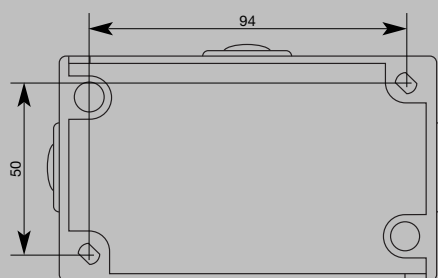
Felfogatócsavarok közötti távolság
