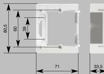
Kiemelő sorolókeret
