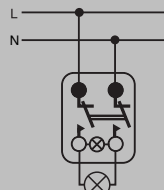
Egypólusú kontroll kapcsoló
