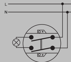
Órás nyomó 12010701, 12010801, 13011401, 13011501
