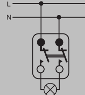
Kétpólusú kapcsoló
