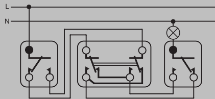
Váltó, alternatív kapcsolás
