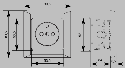
Középföldeléses csatlakozó aljzat
