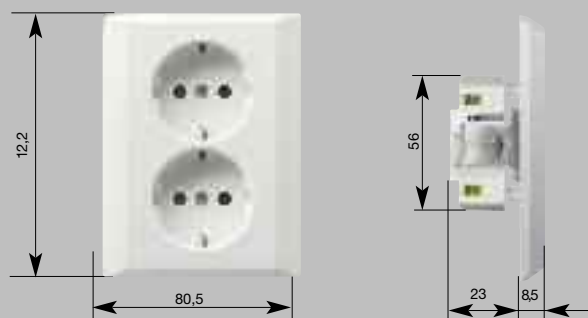
Kettős földelt dugalj
