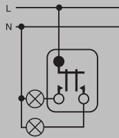
Csillár kapcsoló
