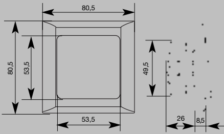
Egypólusú kapcsoló 6
