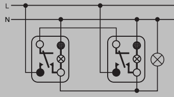
Alternatív kontroll kapcsolás
