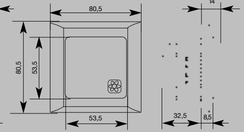
Érintős fényerőszabályzó
