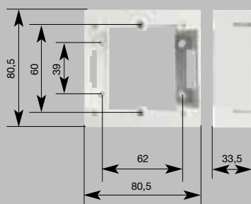
Kiemelő alapteret
