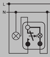
Kontroll nyomó
