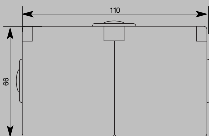
Kettős földelt dugalj
