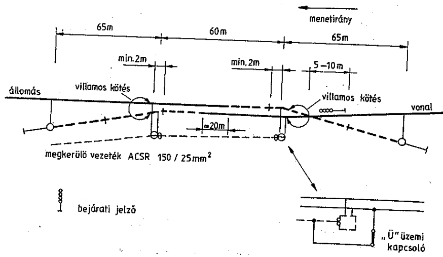
6. ábra Villamos szakaszolás
