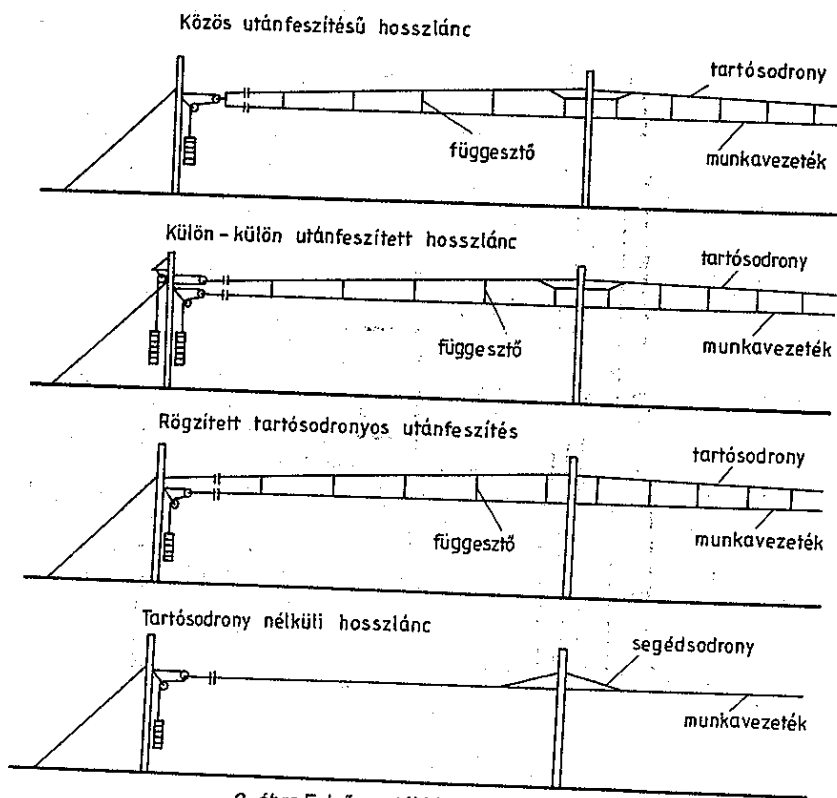
2. ábra Felsővezetéki hosszlánc típusok
