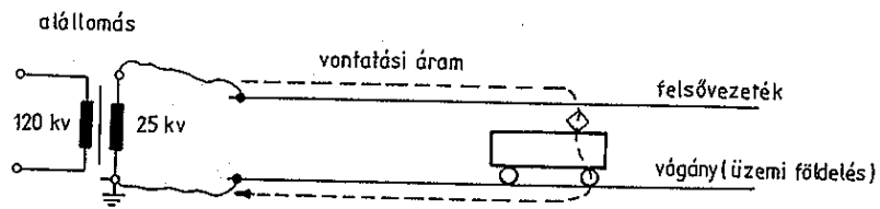
12. ábra A vontatási áram útja
