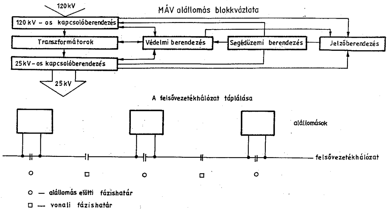
1. ábra MÁV-alállomás blokkvázlata
