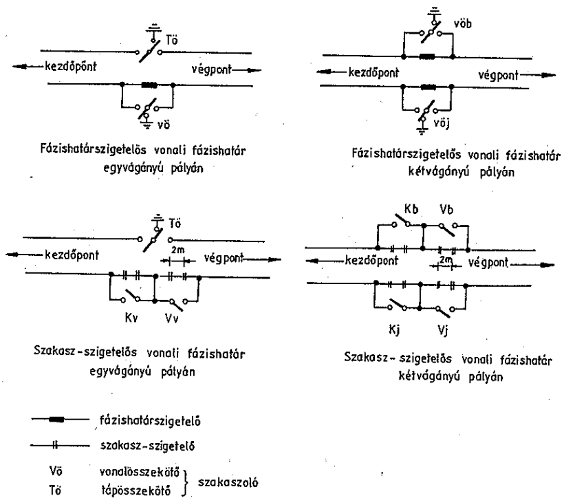
9. ábra Fázishatár-kialakítás szakaszszigetelőkkel
