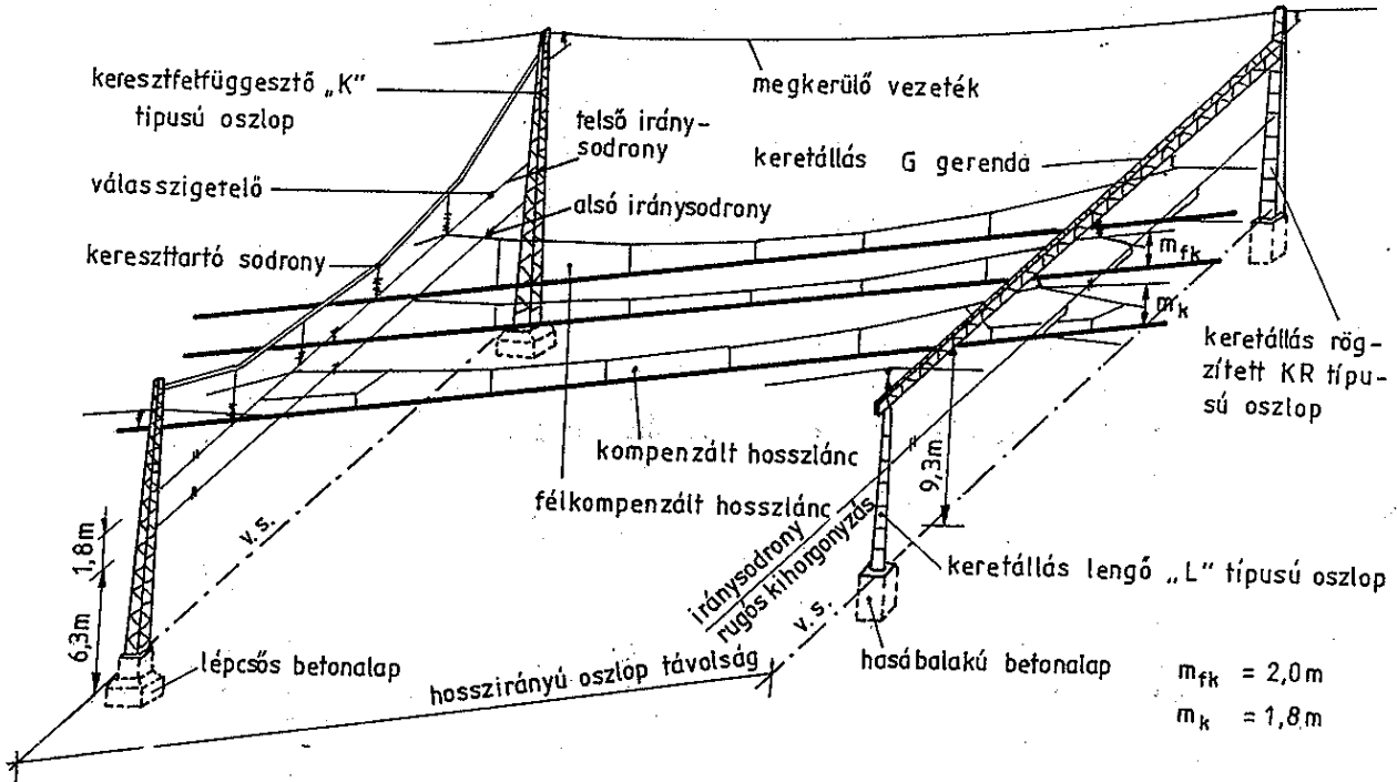
10. ábra Állomási felsővezetési rendszerek
