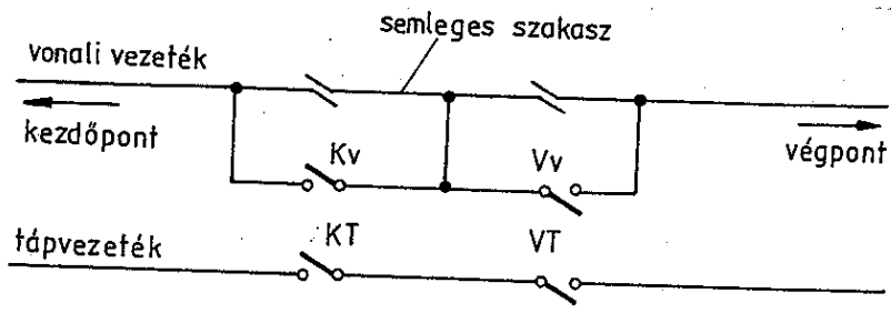
Vonali fázishatár egyvágányú pályán
