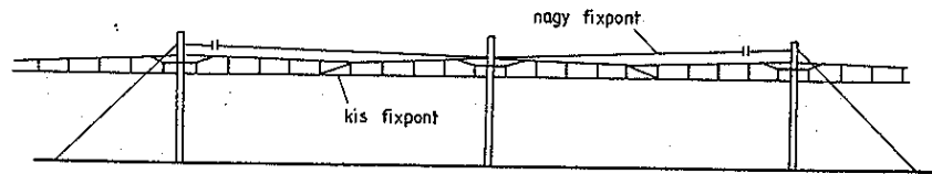
3 ábra A hosszláncok rögzítése
