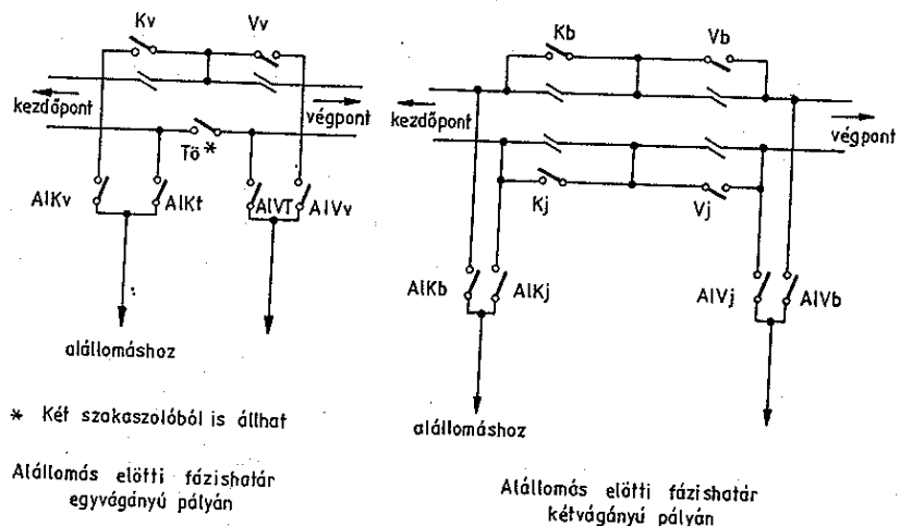
8. ábra Alállomás előtti fázishatárok
