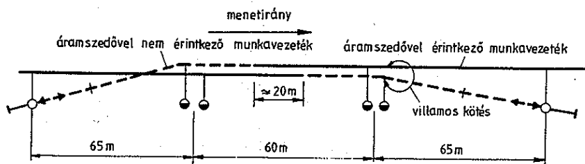
5. ábra Mechanikai szakaszolás
