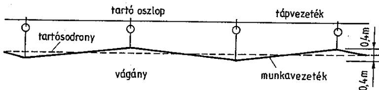
4. ábra Tartószerkezetek, vezetékkigyózás
