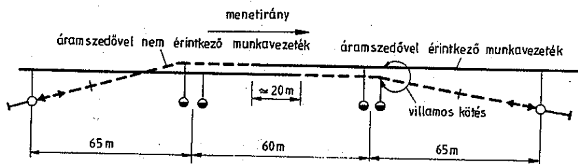
5. ábra Mechanikai szakaszolás
