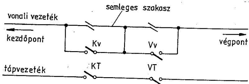
Vonali fázishatár egyvágányú pályán
