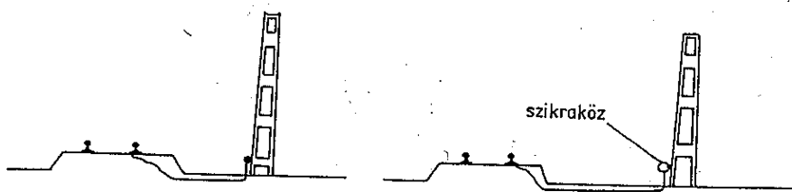
14. ábra Érintésvédelmi földelések
