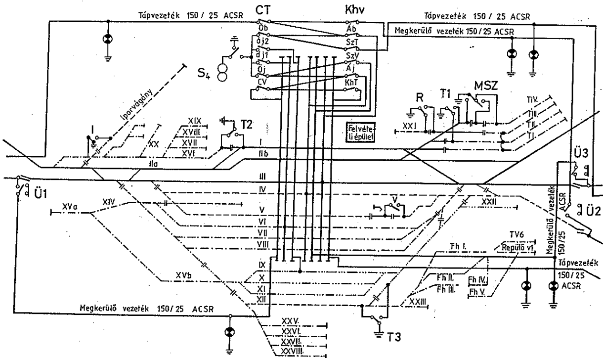
11. ábra Állomási áramkörök
