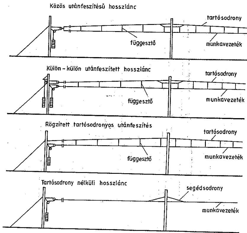
2. ábra Felsővezeték-hálózati hosszlánc típusok
