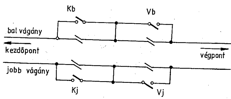
Vonali fázishatár kétvágányú pályán
