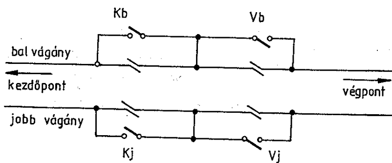
Vonali fázishatár kétvágányú pályán
