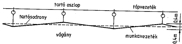
4. ábra Tartószerkezetek, vezetékigyzás
