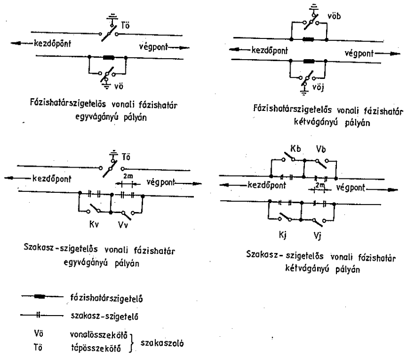
9. ábra Fázishatár-kialaktás szakaszszigetelőkkel
