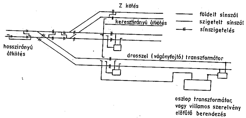
13. ábra Üzemi földelések
