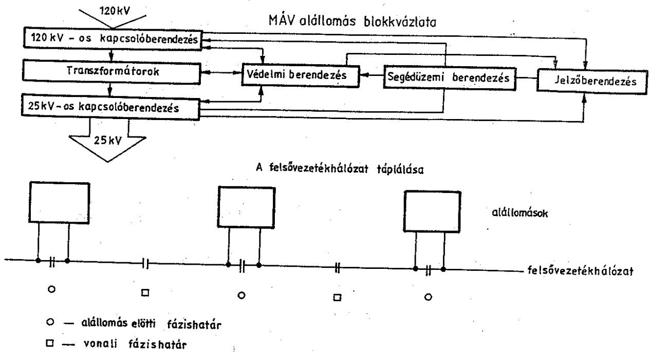
1. ábra MÁV-állomás blokkvázlata
