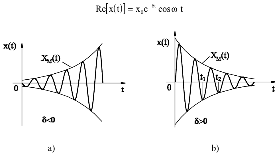
2.8. ábra: Gerjesztett (a) ill. csillapított (b) lengés
