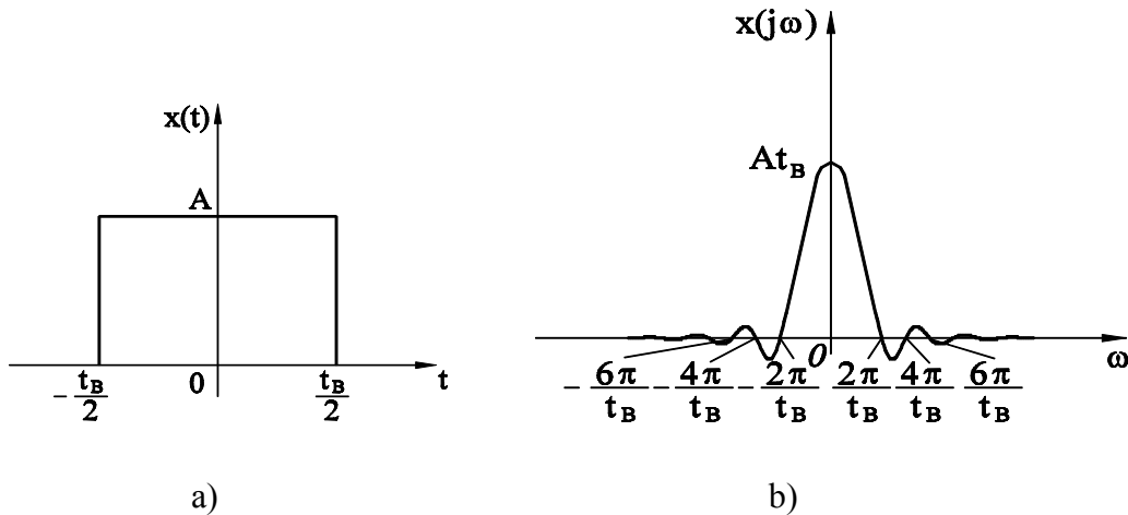
2.11. ábra: A négyzetimpulzus függvénye és Fourier-transzformáltja
