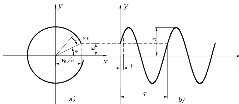
4.3.ábra. A harmonikus lengőmozgás kinematikai jellemzői forgó vektorral is szemléltethetők.
