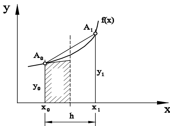
7.2. ábra. Trapézsabály
