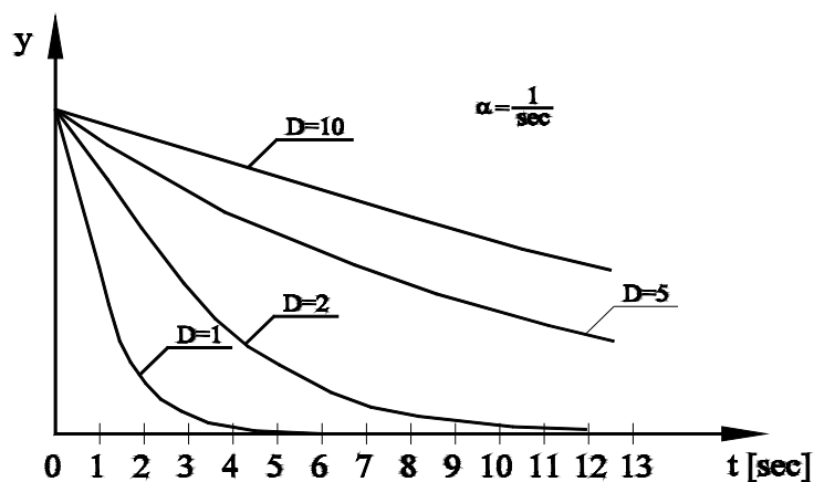
6.1. ábra: A kritikusnál nagyobb csillapítás esetében a mozgás már nem nevezhető lengésnek
