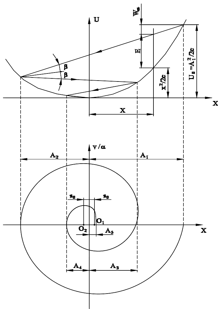
6.6. ábra: Coulomb-féle súrlódás esetében a fázis-görbe félkörívekből áll
