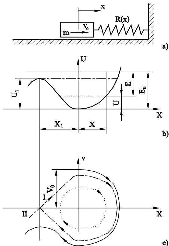
6.5. ábra: A v-x síkon megrajzolt fázisportréről a vizsgált lengőrendszer számos tulajdonsága leolvasható
