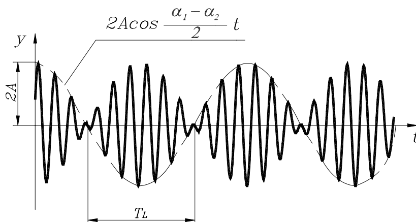
4.4. ábra. Ha a két harmonikus összetevő körfrekvenciája csak kevésbé tér el egymástól, lebegés jön létre.
