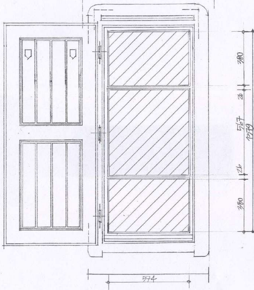
ABLAK HOMLOKZATI NÉZETE M=1:10 ÜZTÖBORDA
