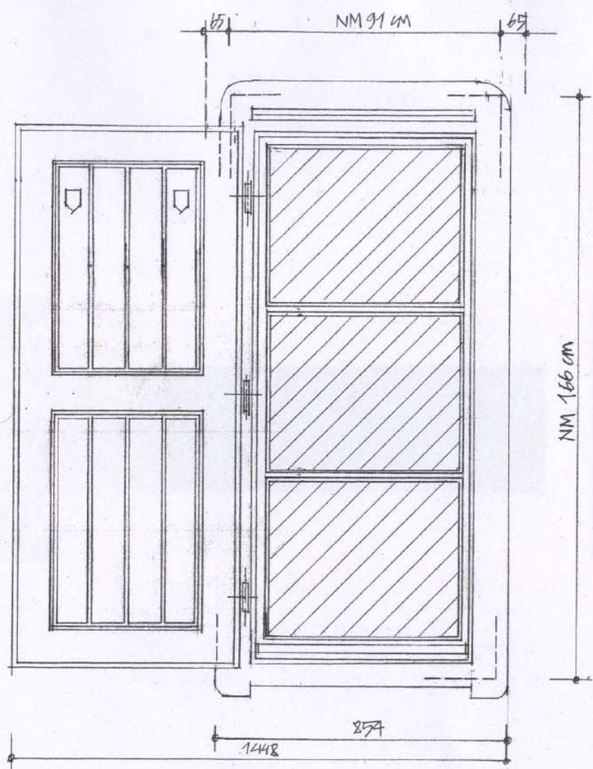
ABLAK HOMLOKZATI NÉZETE M=1:10
