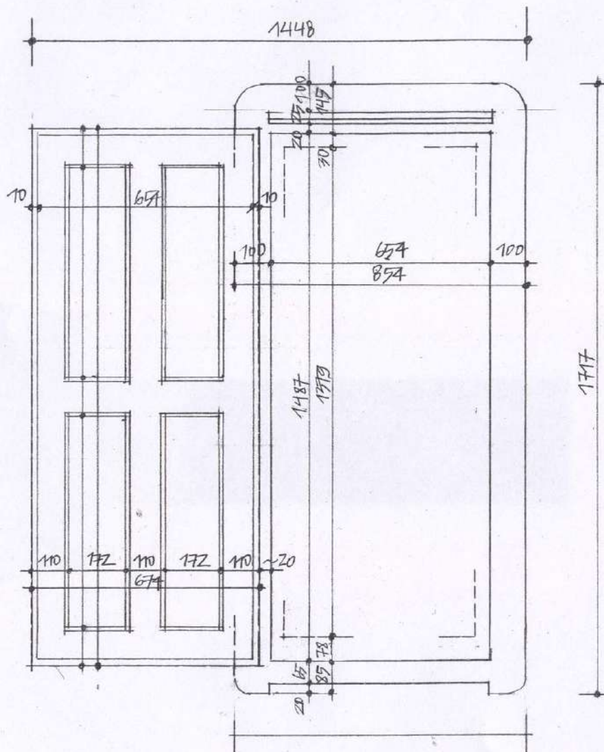
KERET ÉS SPALETTA M=1:10
