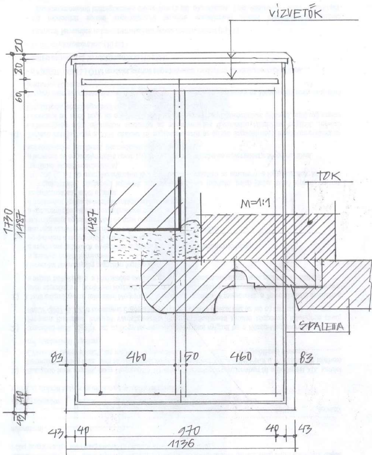
TOKBORÍTÓ KERET M=1:10
